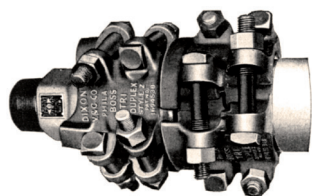
Coupleur Rotatif pour Flexible.
