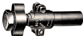
Coupleur Original "Boss".
